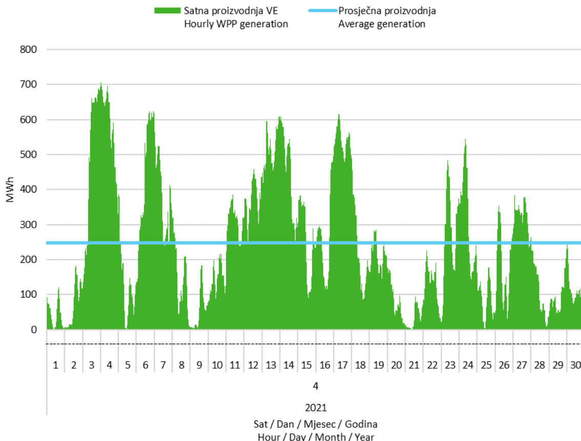
Slika 2 Satna proizvodnja svih vjetroelektrana u travnju 2021. godine
