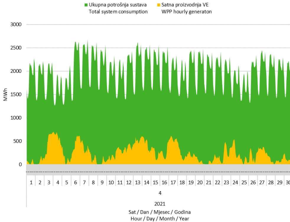
Slika 7 Usporedba satnog dijagrama opterećenja sustava i proizvodnje vjetroelektrana u travnju 2021. godine
