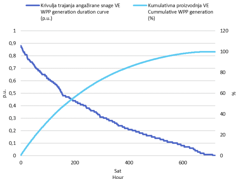
Slika 3 Krivulja trajanja angažirane snage svih VE i kumulativna proizvodnja VE u travnju 2021. godine u jediničnim vrijednostima
