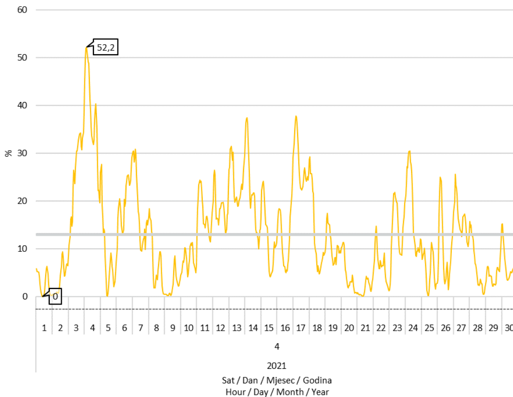
Slika 8 Udio proizvodnje vjetroelektrana u pokrivanju satnog opterećenja elektroenergetskog sustava u travnju 2021. godine
