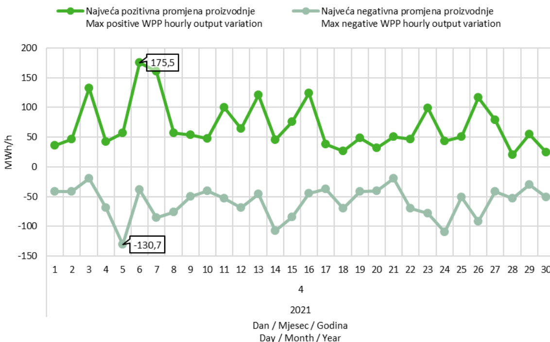
Slika 9 Maksimalna pozitivna i maksimalna negativna promjena satne proizvodnje VE u travnju 2021. godine
