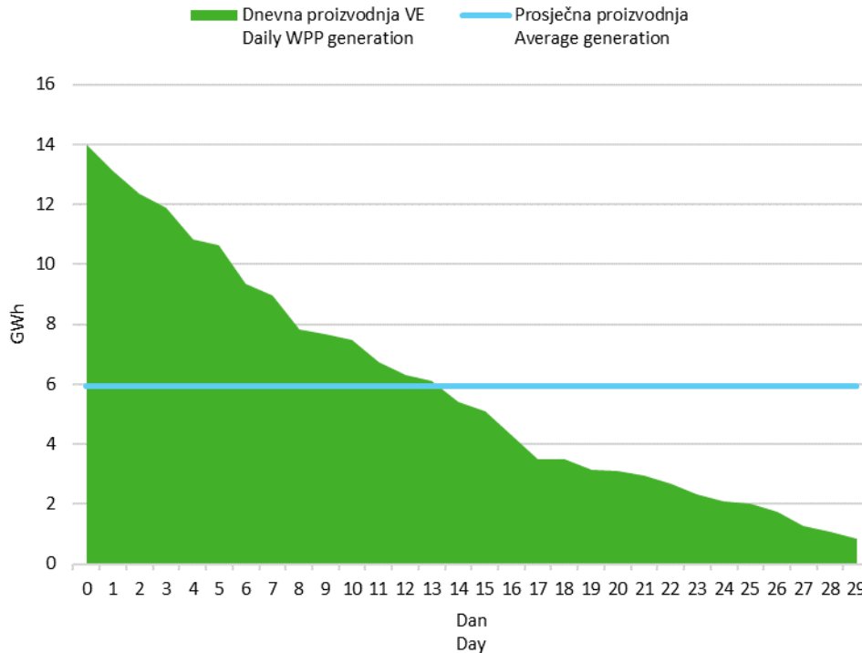
Slika 6 Krivulja trajanja dnevne proizvodnje vjetroelektrana u travnju 2021. godine
