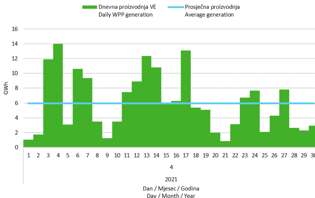
Slika 5 Dnevna proizvodnja svih vjetroelektrana u travnju 2021. godine Figure 5 Daily generation of all wind power plants in April 2021
