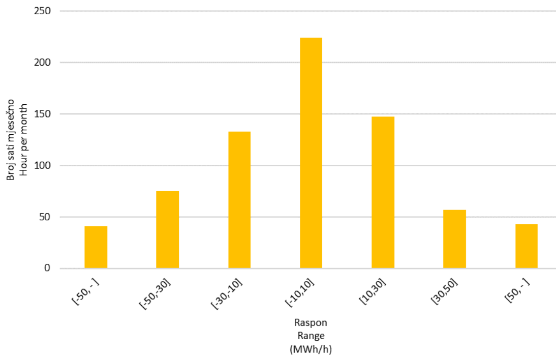
Slika 10 Statistička raspodjela satnih promjena proizvodnje VE u travnju 2021. godine
